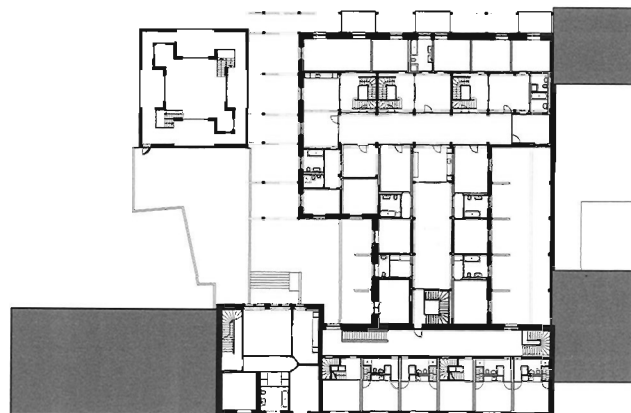
Neubau, 1. Obergeschoss
