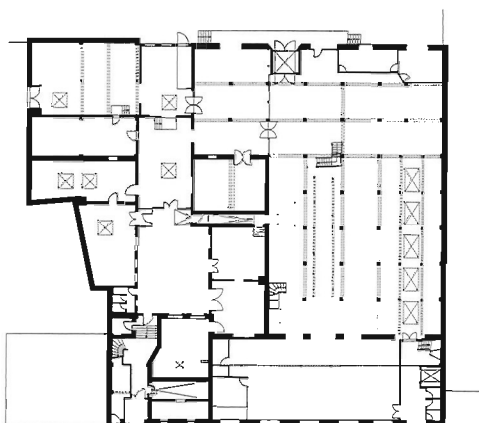
Bestand, Erdgeschoss
